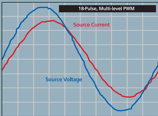
罗宾康完美无谐波系列波形
