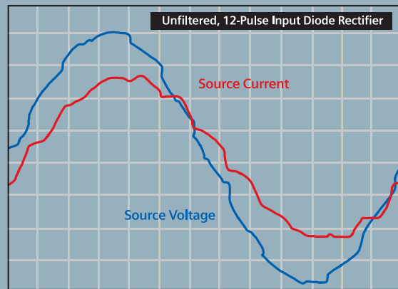
12 脉冲谐波波形
